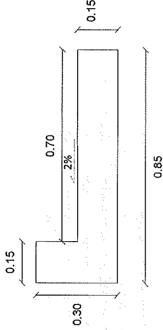
Croquis ejecucion de cordon cuneta.
