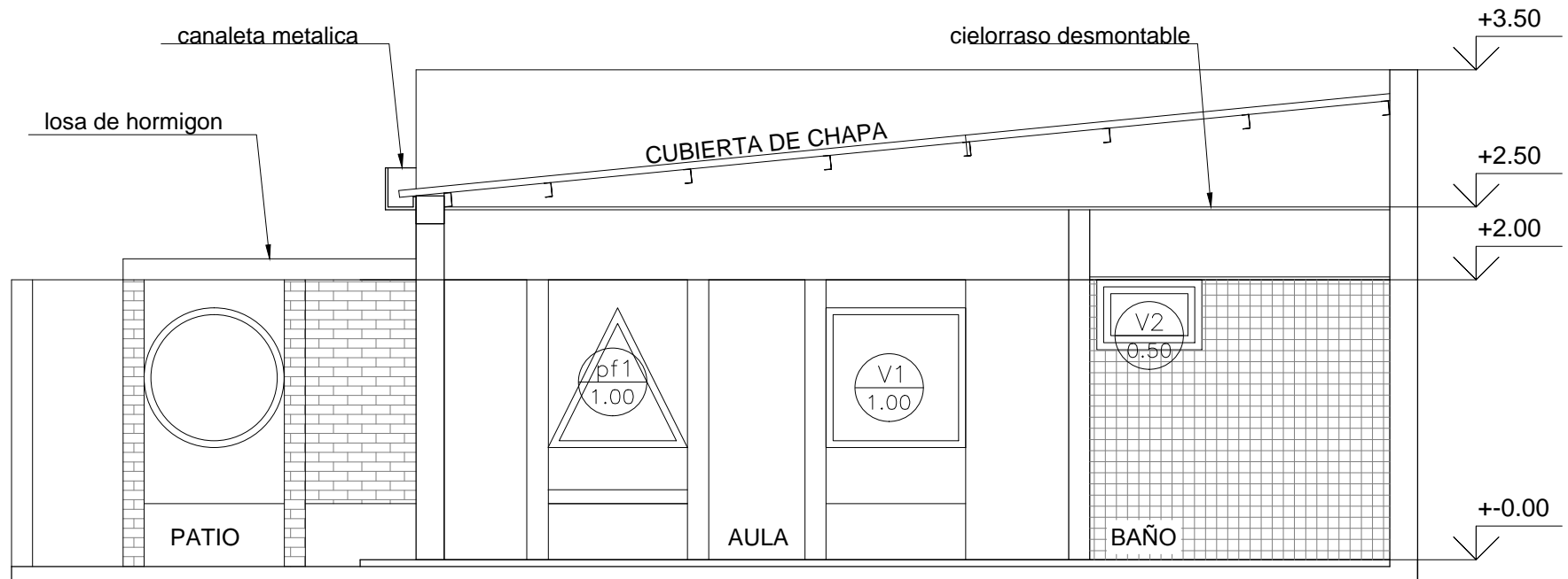
corte A-A
