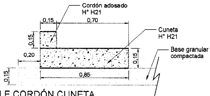
DETALLE CORDÓN CUNETA ESC: 1:20
